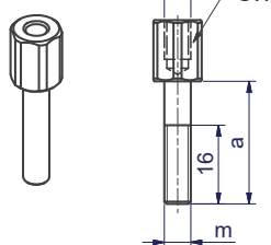
DIN 938
