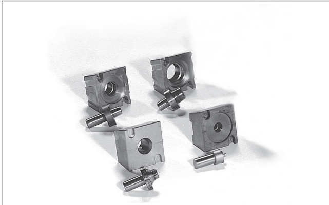
Parflange® tools
